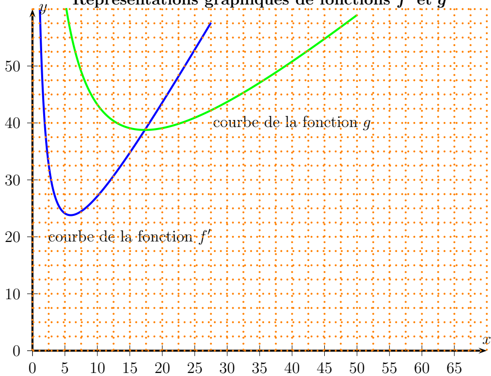
Représentations graphiques de fonctions f' et g
