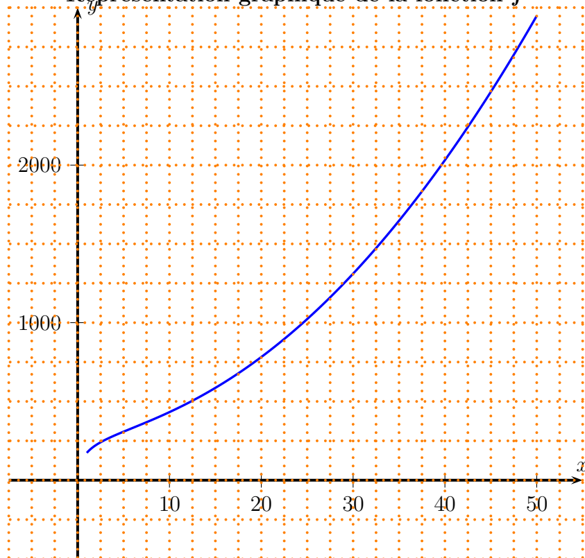
Représentation graphique de la fonction f
